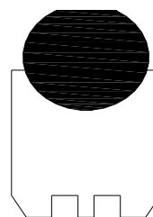
Trade name: Turcon® Roto Glyd Ring® Figure No.7.36 (d)
